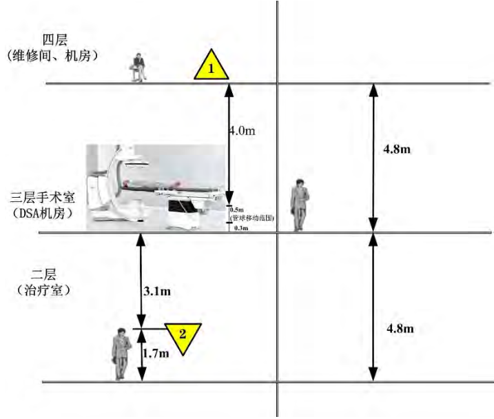
图 11-7 DSA 手术室估算点位置剖面示意图
