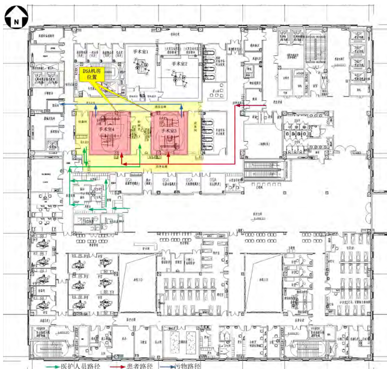
图 11-1 平急两用综合楼地上三层局部布局及 DSA 手术室位置和路由示意图
