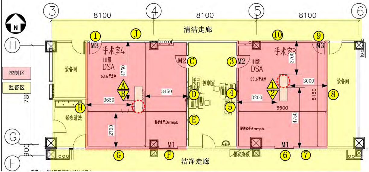
图 11-6 DSA 手术室估算点位置平面示意图
