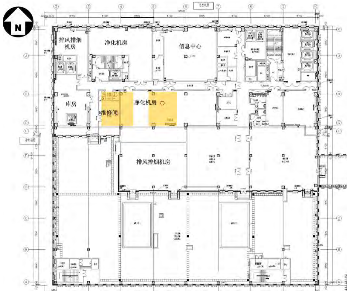
图 7-4 平急两用综合楼地上四层布局以及新建 DSA 手术室对应位置示意图
