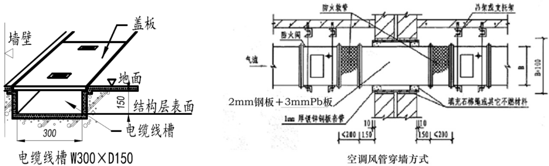
图 10-1 DSA 机房电缆和空调风管穿墙方式示意图
