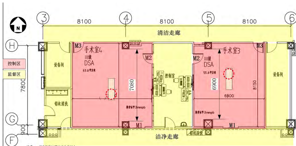
图 11-2 本项目新建 DSA 场所布局示意图
